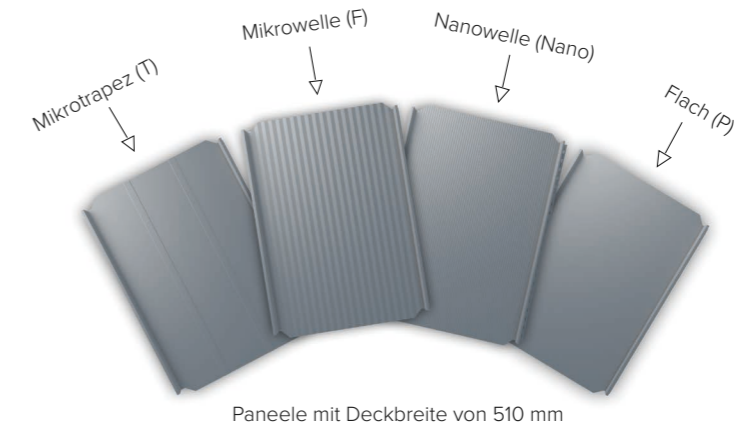
Paneele mit Deckbreite von 510 mm
