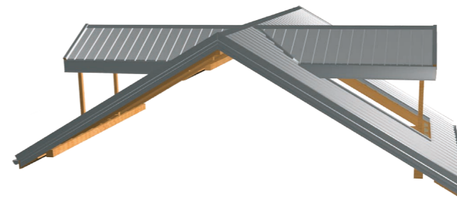
ABB. 25 Spitzen-Kantenteile – Windfedern
