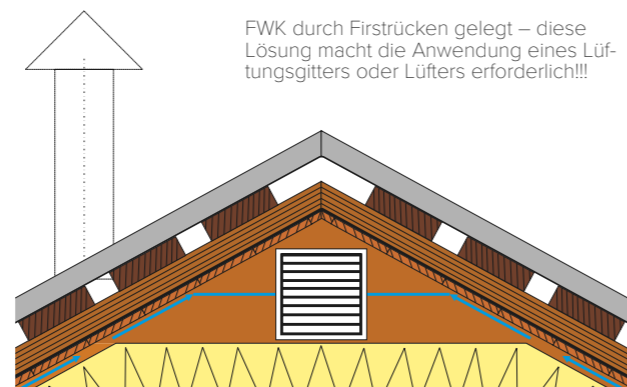
ABB. 6 Beispiellösungen die Traufe- und First-Linie – verschaltes Dach + Pappe
