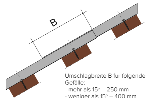
ABB. 21 Umschlagbreite – B
