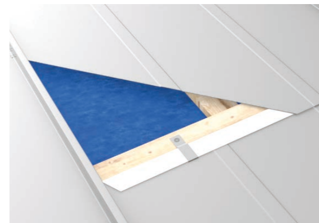
ABB. 15 Paneel-Verbindung durch Biegen
